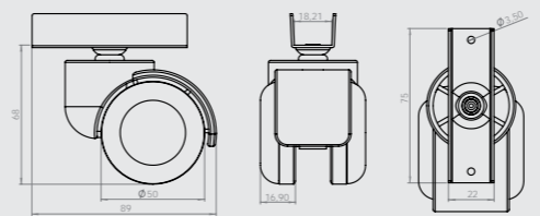
454 Büro Krom Gövdeli Uzun U-Tablalı Bureau Chrome Body Long U-shape Board Caster Бюро Ролик с Хромированным Корпусом и Длинной U-образной Планкой
