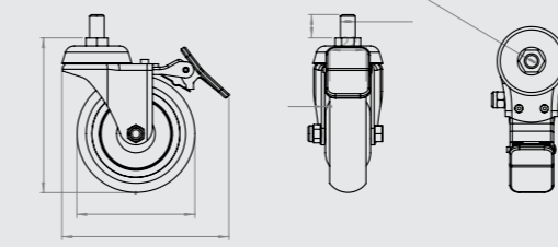
664 125'lik Market Tipi Vidalı Frenli 125mm Market Type Screwed Caster with Brake 125мм Маркет Типный Ролик с Винтом и Тормозом
