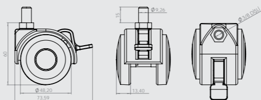
426 Plastik Gri Büyük Vidalı Frenli Plastic Grey Big Screwed Caster with Brake Пластиковый Серый Ролик с Большой Винтом и Тормозом
