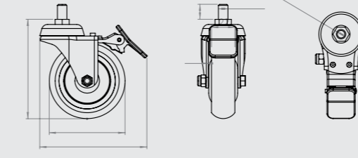
654 100'lük Market Tipi Vidalı Frenli 100mm Market Type Screwed Caster with Brake 100мм Маркет Типный Ролик с Винтом и Тормозом
