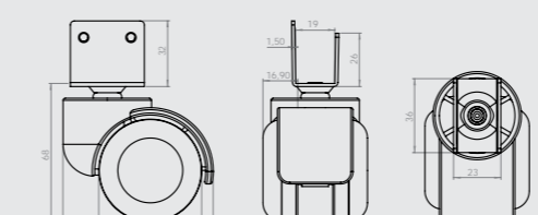
455 Büro Krom gövdeli kısa U-Tablalı Bureau Chrome Body Short U-shape Board Caster Бюро Ролик с Хромированным Корпусом и Короткой U-образной Планкой
