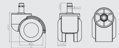
453 Büro Krom Gövdeli Kalın Pimli Bureau Chrome Body Thick Pin Caster Бюро ролик с Хромированным корпусом и Толстым Штырем
