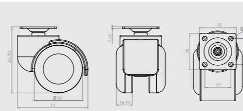
451 Büro Krom Gövdeli Tablalı Bureau Chrome Body Board Caster Бюро ролик с Хромированным корпусом и Планкой
