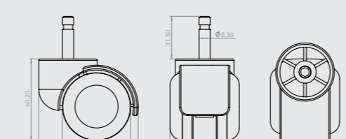
456 Büro Krom Gövdeli İnce Pimli Bureau Chrome Body Thin Pin Caster Бюро Ролик с Хромированным Корпусом Тонким Штырем
