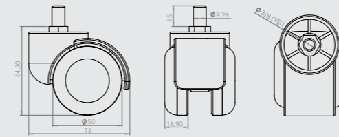
452 Büro Krom Gövdeli Vidalı Bureau Chrome Body Screwed Caster Бюро ролик с Хромированным корпусом и Винтом
