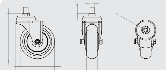
662 125'lik Market Tipi Vidalı 125mm Market Type Screwed Caster 125мм Маркет Типный Ролик с Винтом
