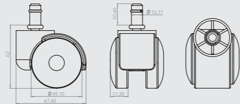
419 Büro Tipi Gri Kalın Pimli Bureau Type Grey Thick Pin Caster Бюро Типный Серый Ролик с Толстым Штырем
